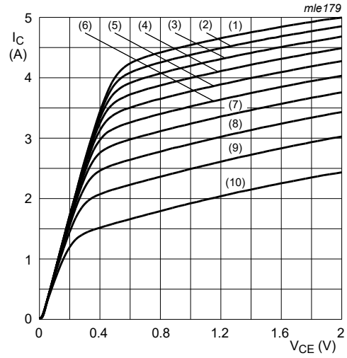
T_{amb} = 25\text{ }^\circ\text{C} (1) I_B = 120\text{ mA} (2) I_B = 108\text{ mA} (3) I_B = 96\text{ mA} (4) I_B = 84\text{ mA} (5) I_B = 72\text{ mA} (6) I_B = 60\text{ mA} (7) I_B = 48\text{ mA} (8) I_B = 36\text{ mA} (9) I_B = 24\text{ mA} (10) I_B = 12\text{ mA}
