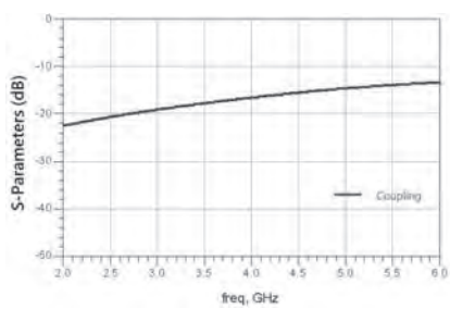
RFCPL1608070P08Q1C
