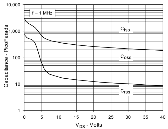
Fig. 10. Capacitance
