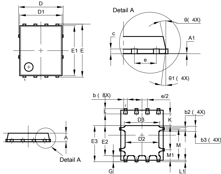
PowerDI5060-8
