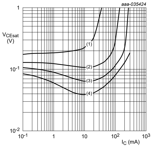
T_{amb} = 25\text{ }^\circ\text{C} (1) I_C/I_B = 50 (2) I_C/I_B = 20 (3) I_C/I_B = 10 (4) I_C/I_B = 5
