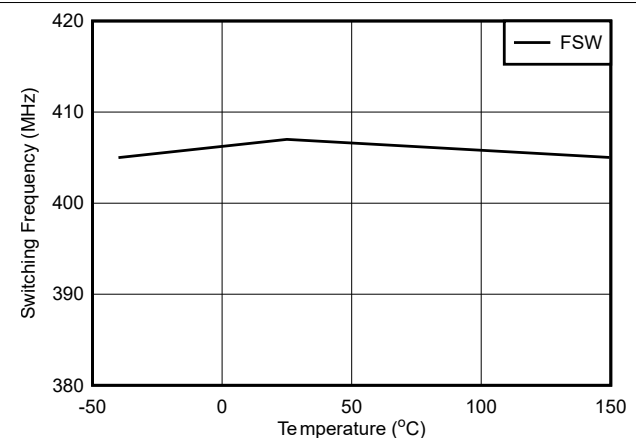
Figure 6-6. f_{SW} 400kHz
