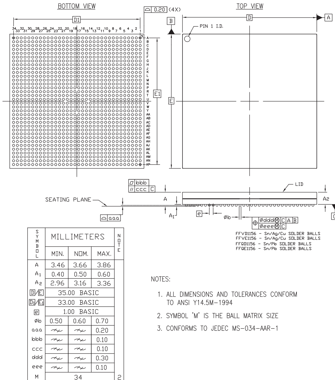
Figure 5-21: Package Dimensions for FFVE1156 (XCZU21DR) and FFVE1156 (XCZU25DR, XCZU27DR, XCZU28DR, XCZU42DR, XCZU43DR, XCZU47DR, XCZU48DR, XCZU63DR, XCZU64DR, XCZU65DR, XCZU67DR)
