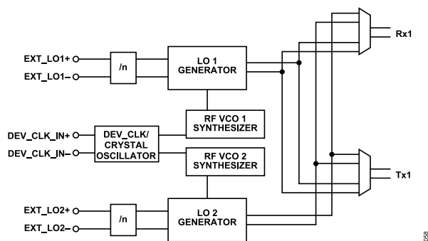
Figure 362. RF LO
