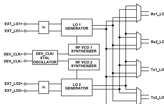
Figure 362. RF LO
