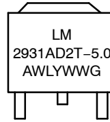
D2PAK D2T SUFFIX CASE 936
