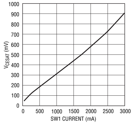
SW1 V_{\text{CESAT}}
