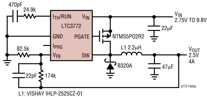
L1: VISHAY IHLP-2525CZ-01
