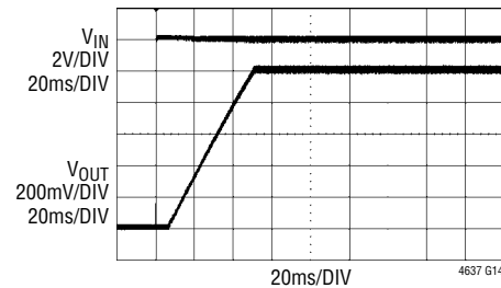
Turn-On 20A Load
