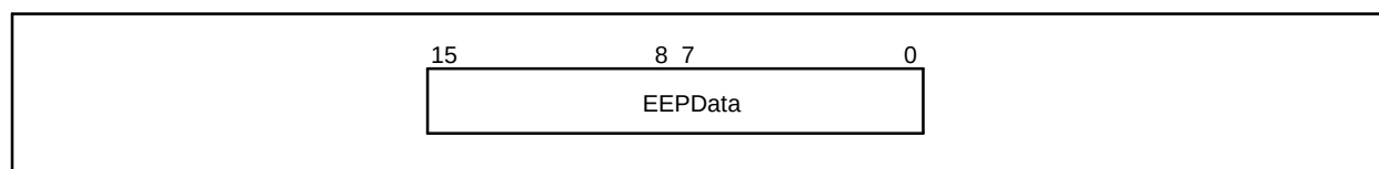
Fig. 7.7 EEPROMData Register Map
