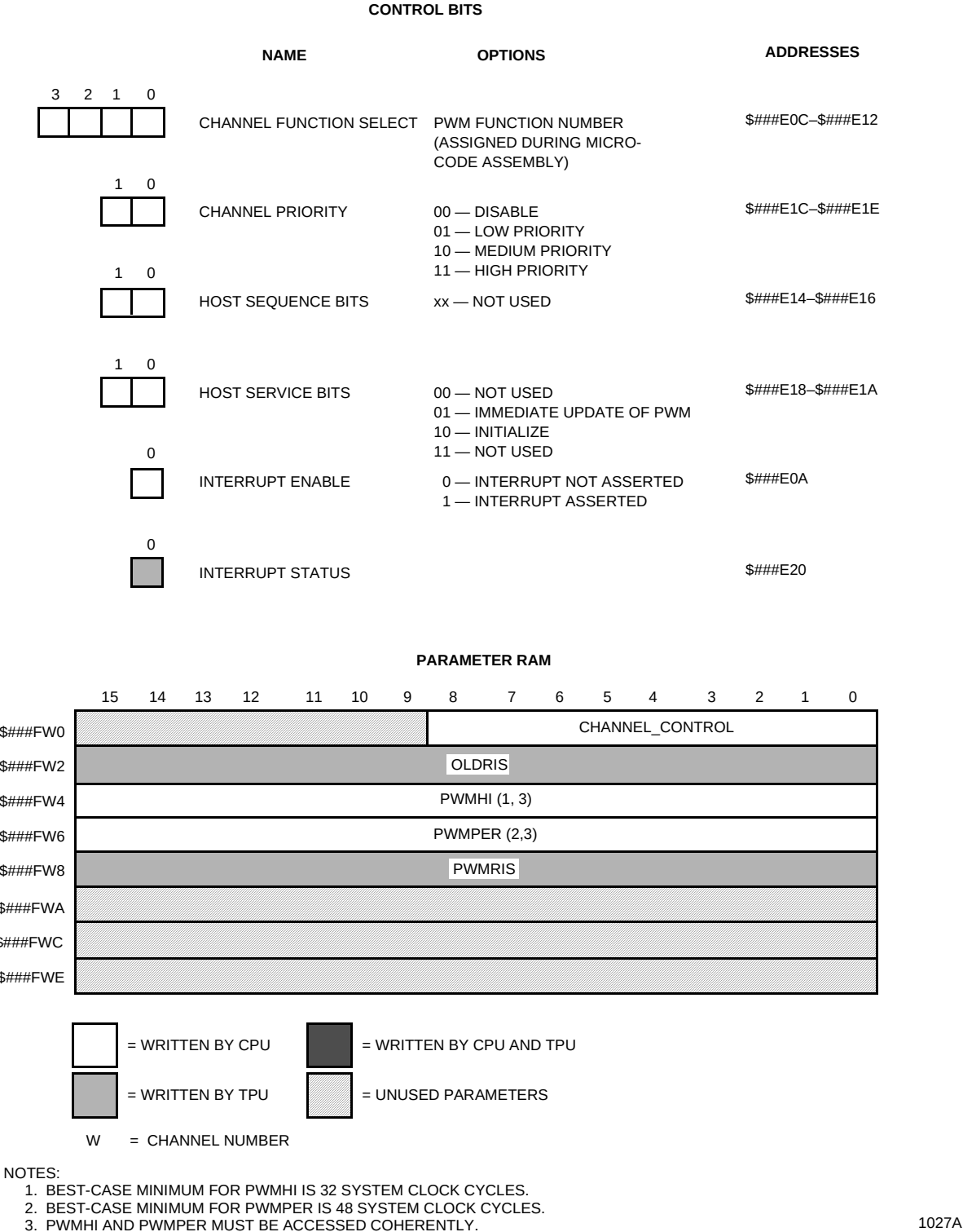
Figure D-23 PWM Parameters
