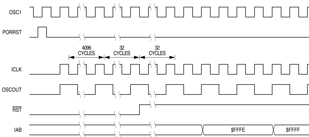
Figure 4-7. POR Recovery
