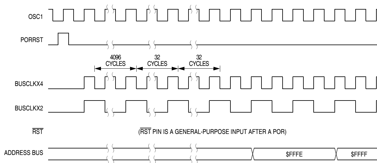
Figure 14-6. POR Recovery
