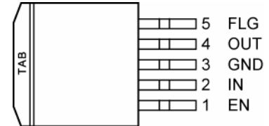
MIC39151-x.xBU/WU TO-263-5 (D 2 Pak) (U)
