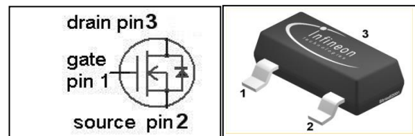
PG-SOT-23
