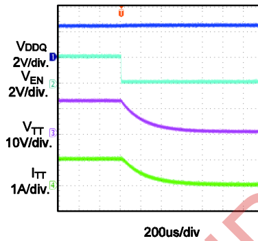
Enable Off
