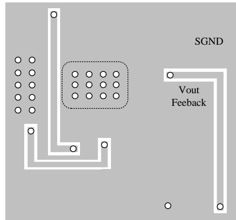
Bottom Layer
