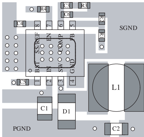
Top Layer
