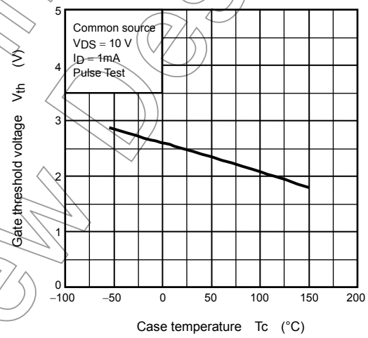
V_{th} - T_c
