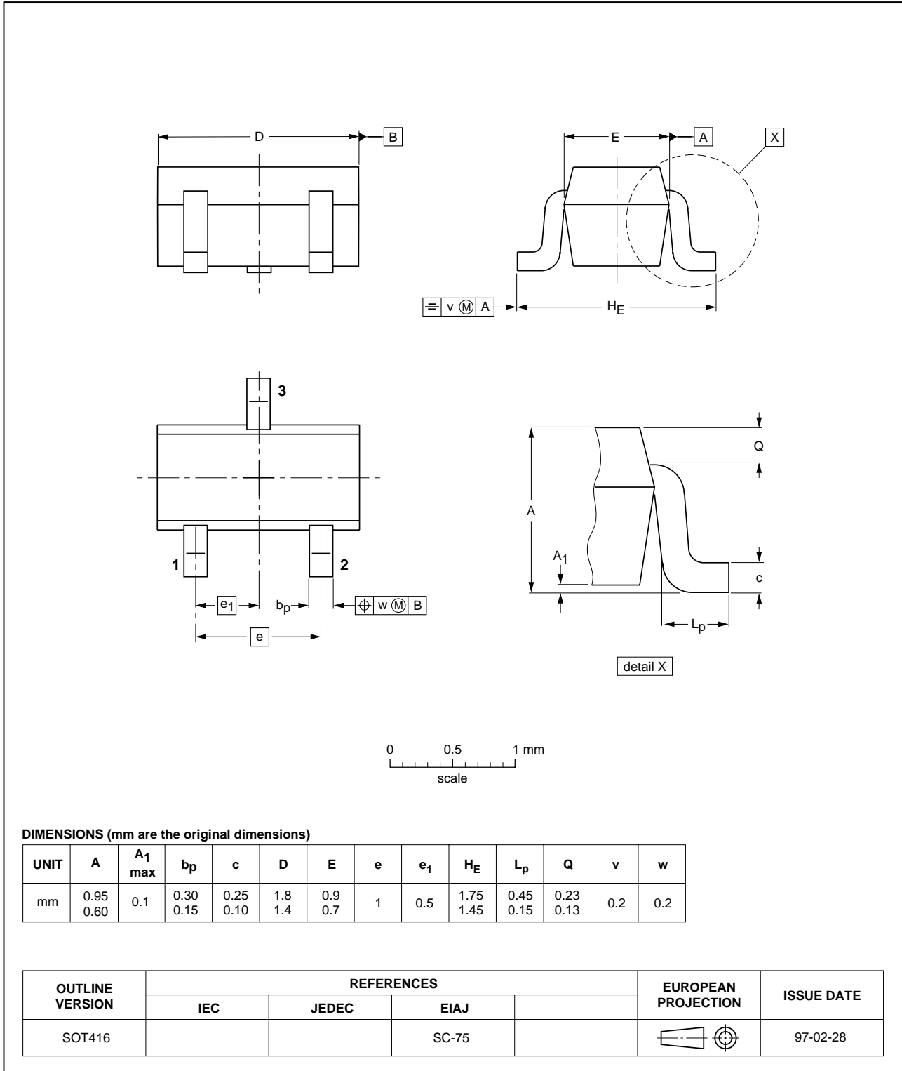
Fig 14. SOT416 (SC-75).
