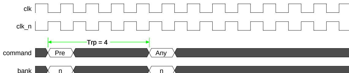
Figure 14: Trp Timing Parameter
