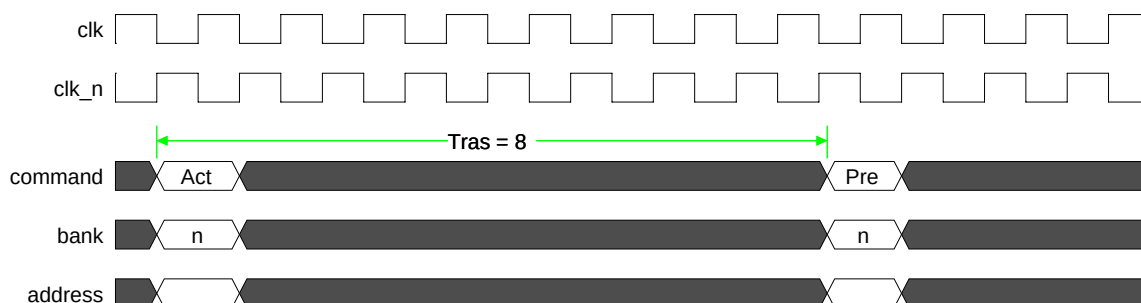
Figure 13: Tras Timing Parameter
