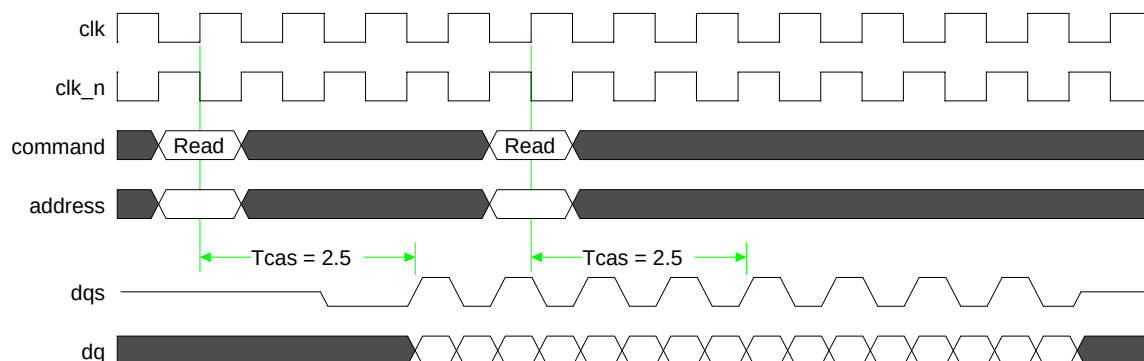
Figure 9: Tcas Timing Parameter
