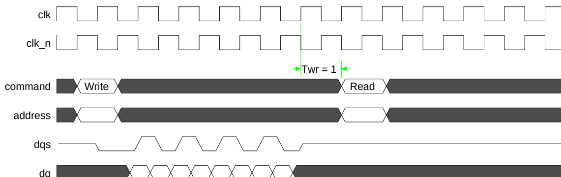
Figure 12: Twr Timing Parameter
