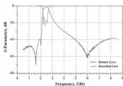
RFBPF2012080A6T
