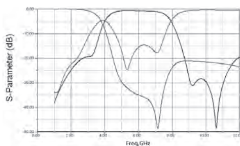
RFDIP2012050LQT
