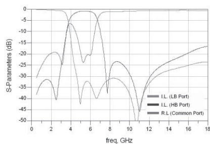
RFDIP1606L21T
