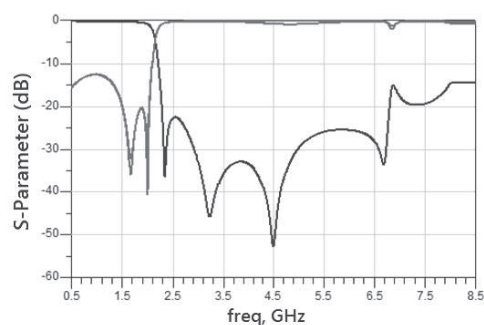
RFLPF3225100Q07B1U
