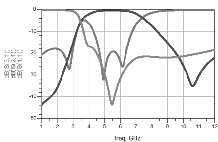
RFDIP2012050LWT
