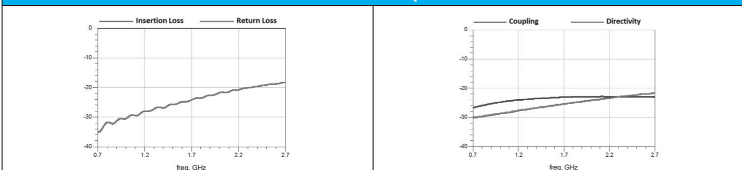
RFCPL1608070P28Q1C
