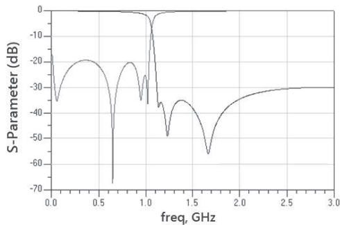
RFLPF3225100Q07B1U
