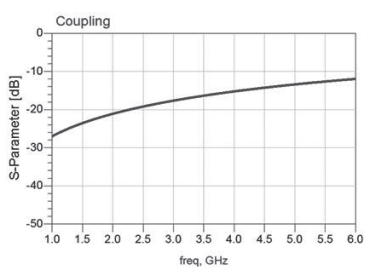
RFCPL0605030L58Q1C
