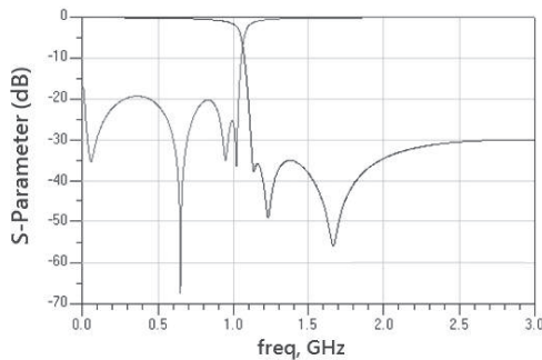
RFLPF3225100Q07B1U
