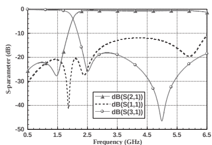
RFDIP1608060TAT
