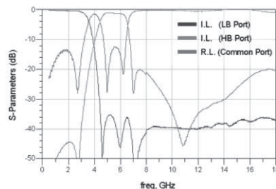
RFDIP1606L29T
