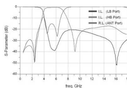
RFDIP1608060LY8Q1C
