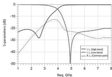
RFDIP1606L24T
