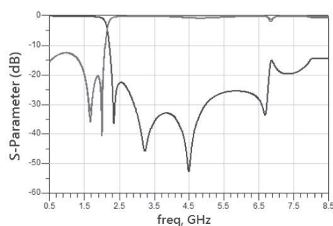
RFLPF3225100Q07B1U
