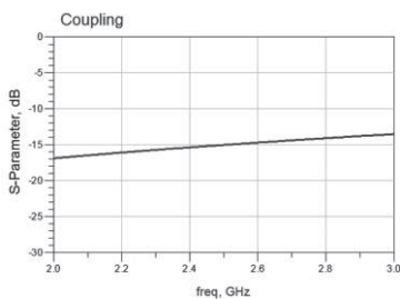
FCPL0605030L28Q1C
