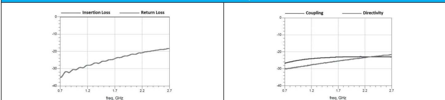
RFCPL1608070P18Q1C
