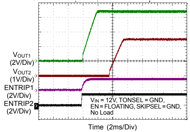
VOUT1 Delay-Start
