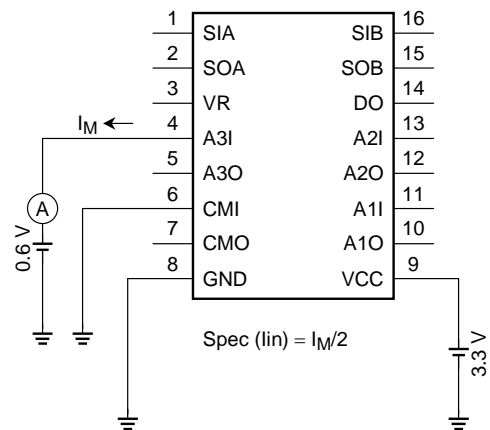
(14) OP-AMP3
