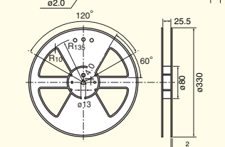
Reel dimensions
