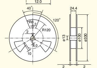
Reel dimensions
