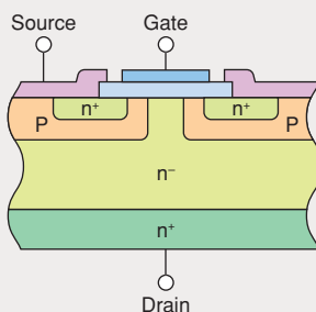
Double-Diffusion Structure
