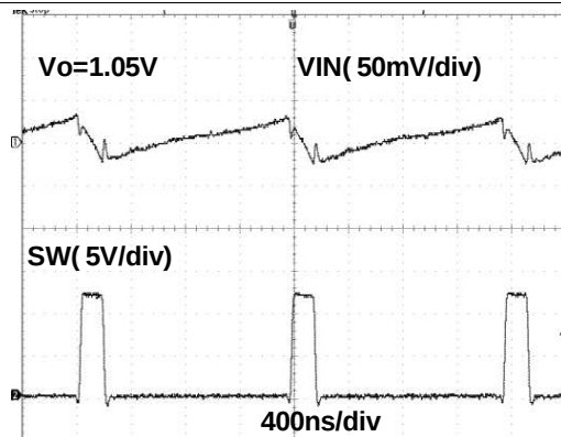
Figure 15. VIN Ripple
