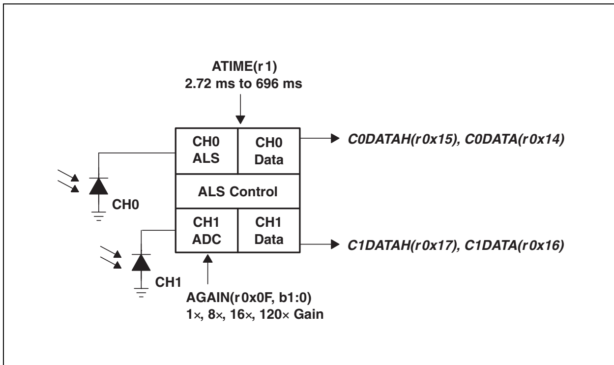
Figure 18: ALS Operation
