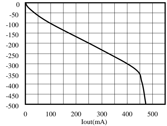
V_{drop}(mV) V_{drop}
