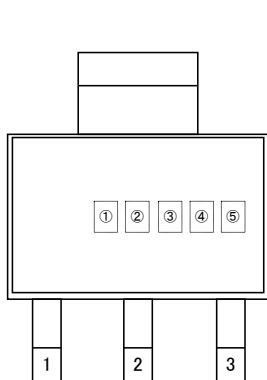
SOT-223
