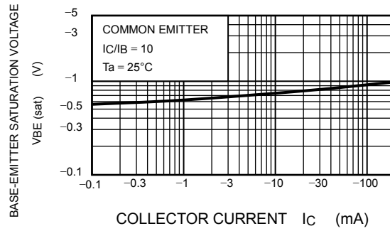
V_{BE(sat)} - I_C
