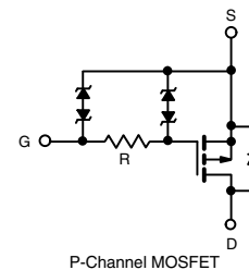
P-Channel MOSFET
