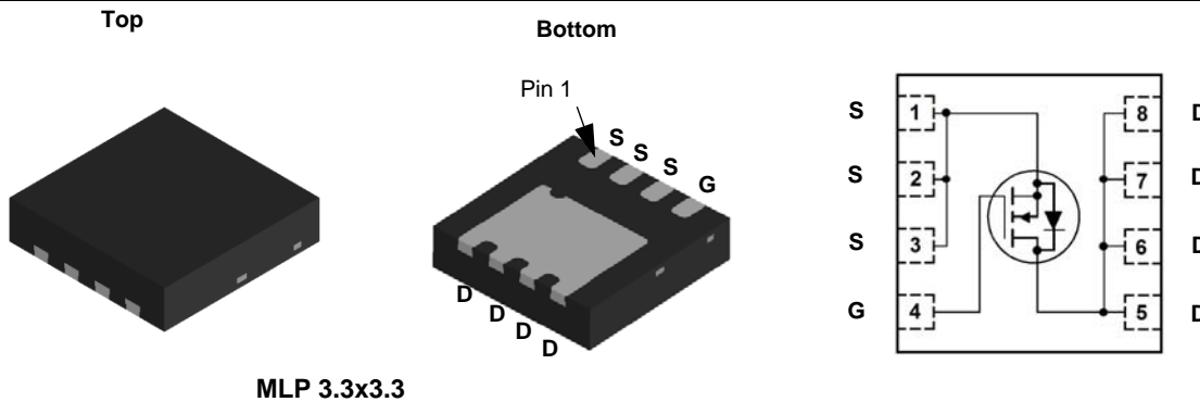
MLP 3.3x3.3
