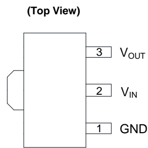
SOT-89 (Option 1)/ R Package
