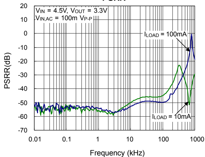
PSRR
