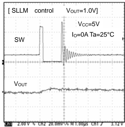
Figure 15. SW Waveform (I O =0mA)
