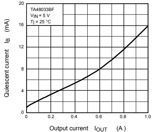
I_B - I_{OUT}
