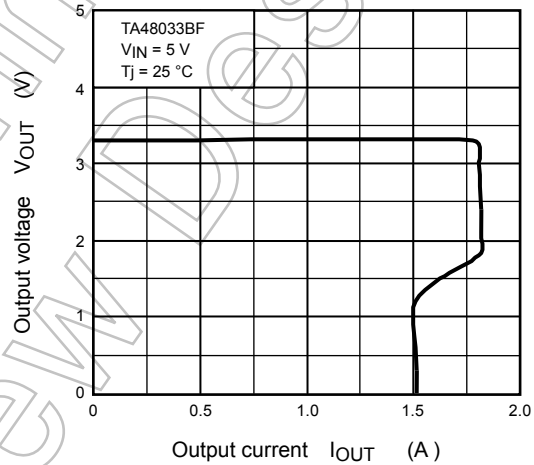
V_{OUT} - I_{OUT}
