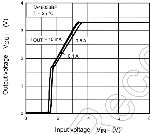
V_{OUT} - V_{IN}
