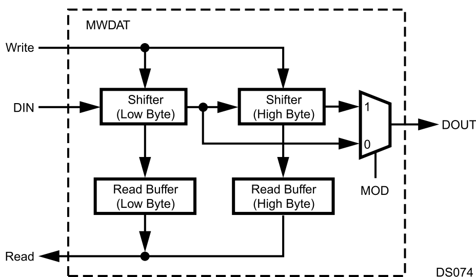
Figure 23-8. MWDAT Register
