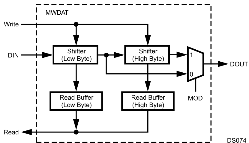
Figure 22-8. MWDAT Register
