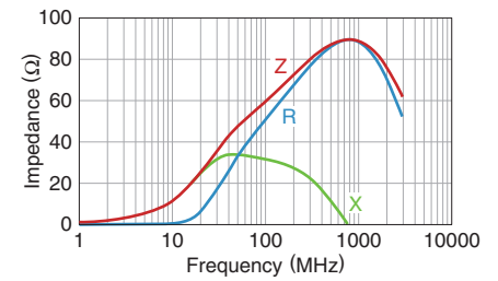
MPZ1005S600CT000
