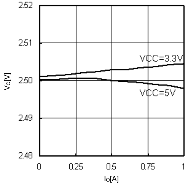
Fig.18 I_o - V_o ( V_o=2.5V )
