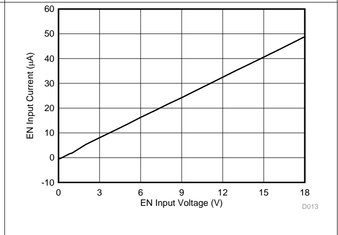
Figure 13. EN Current vs EN Voltage
