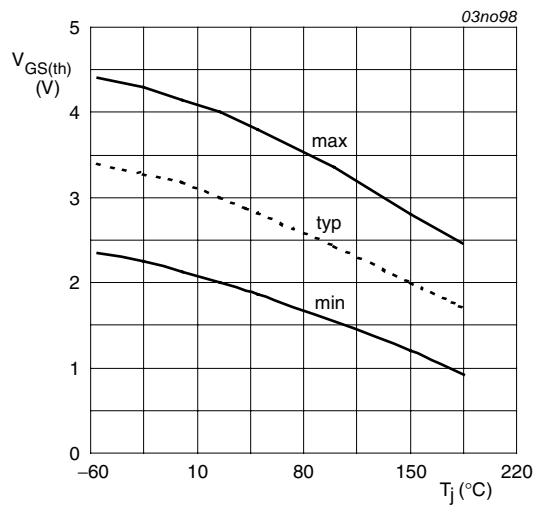
I_D = 1\text{mA}; V_{DS} = V_{GS}
