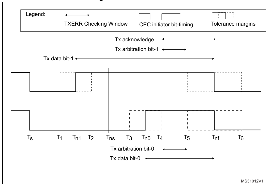
Figure 586. TXERR detection
