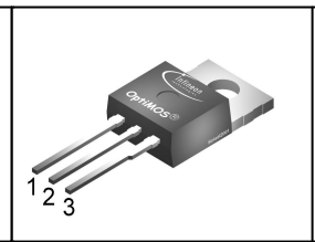
P- TO220 -3-1
