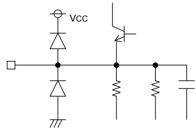
19pin (VREG)
